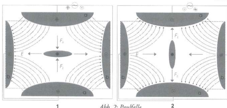
Abb. 2: Paulfalle
