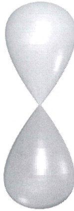
p-Orbital
