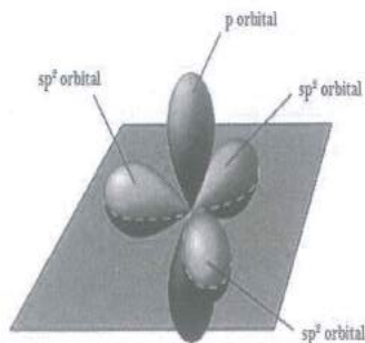
Die Orbitale um ein C-Orbital
